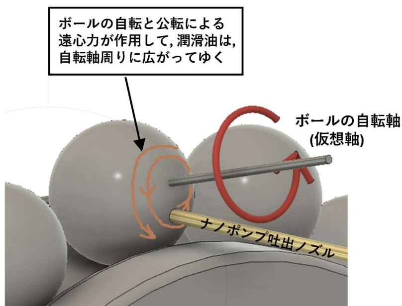
図6 ナノポンプ®によるナノ潤滑の仕組み
